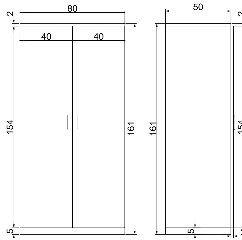
VISTA FRONTAL VISTA LATERAL ESQUERDA PERSPECTIVA ISOMÉTRICA
